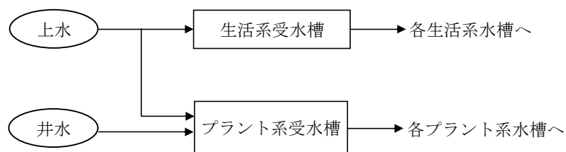
図 2.1 給水フロー（参考）
