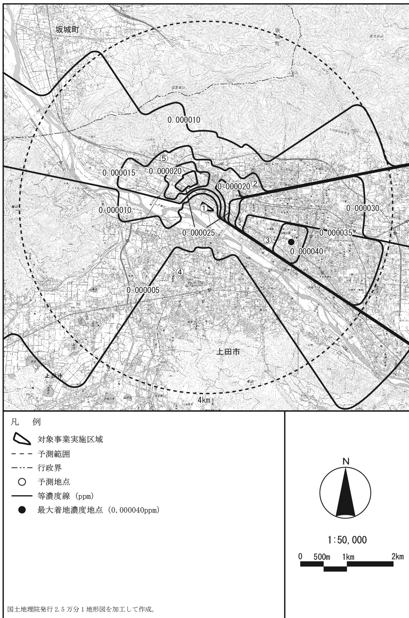
図 4.1-22(2) 年平均値寄与濃度分布予測結果 (二酸化窒素) 1.4-90
