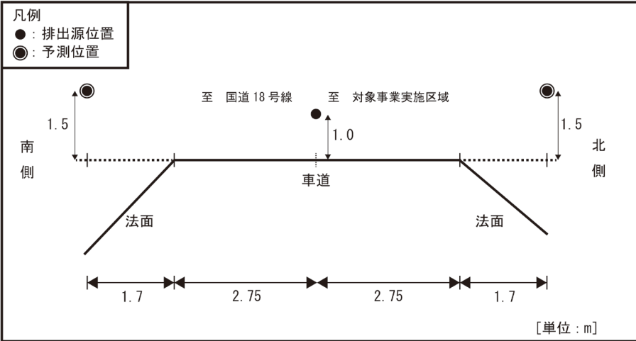
図 4.1-17 予測地点の道路条件、排出源位置
