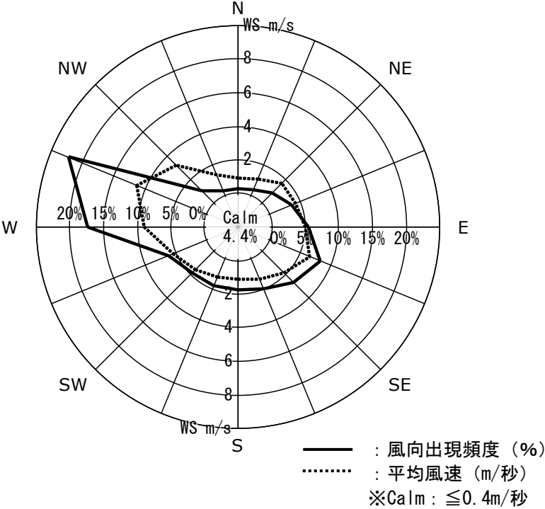
図 4.1-2 年間風配図
