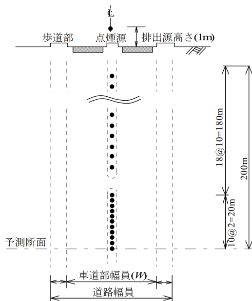
図 4.1-10 点煙源の配置
