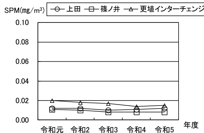
図 2.2-24 浮遊粒子状物質年平均値の経年変化(令和元年度～令和5年度)
