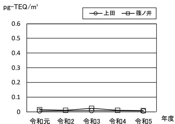
図 2. 2-27 ダイオキシン類の経年変化(令和元年度～令和5年度)
