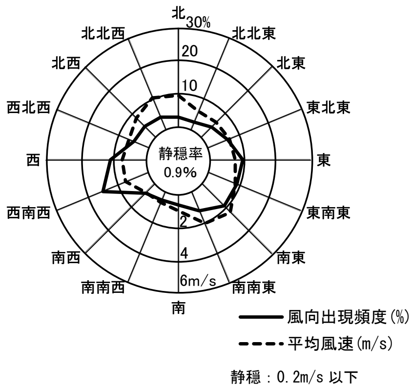
図 2.2-3 上田地域気象観測所における風配図(令和 5 年)
