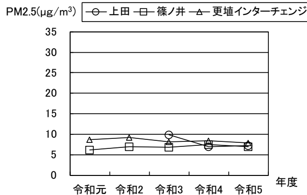
図 2.2-25 微小粒子状物質年平均値の経年変化(令和元年度～令和5年度)
