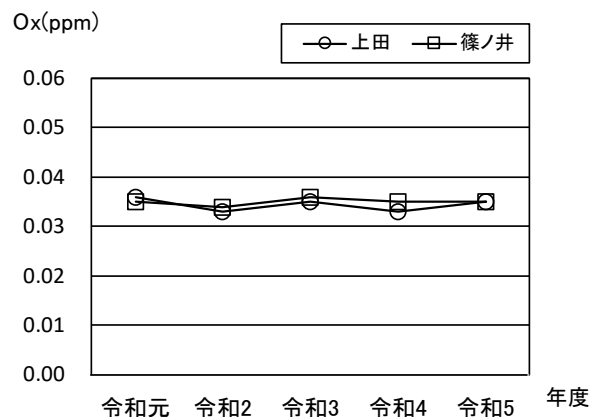
図 2.2-26 光化学オキシダント年平均値の経年変化(令和元年度～令和5年度)
