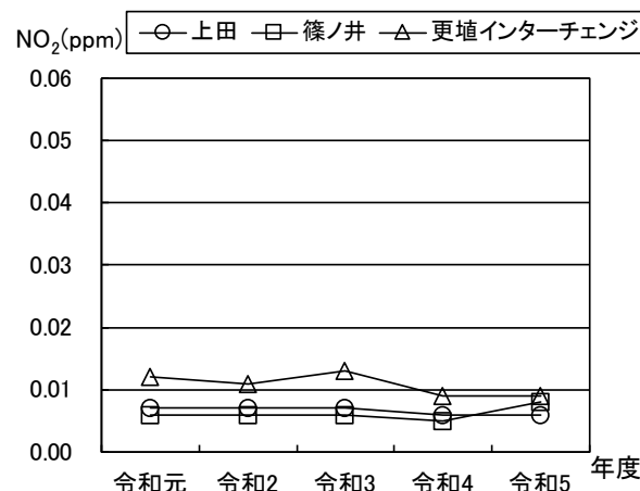
図 2.2-23 二酸化窒素年平均値の経年変化(令和元年度～令和5年度)
