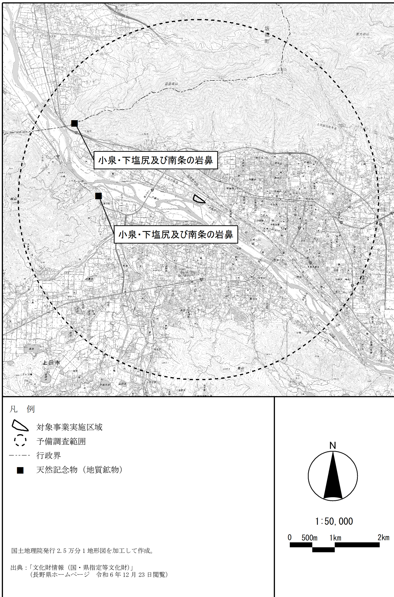
図 2.2-9 対象事業実施区域及びその周囲の天然記念物（地質鉱物）
