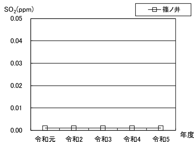
図 2. 2-22 二酸化硫黄年平均値の経年変化(令和元年度～令和5年度)
