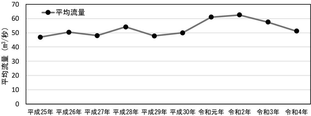
図 2.2-4 生田水文水質観測所における平均流量の推移（平成25年～令和4年）
