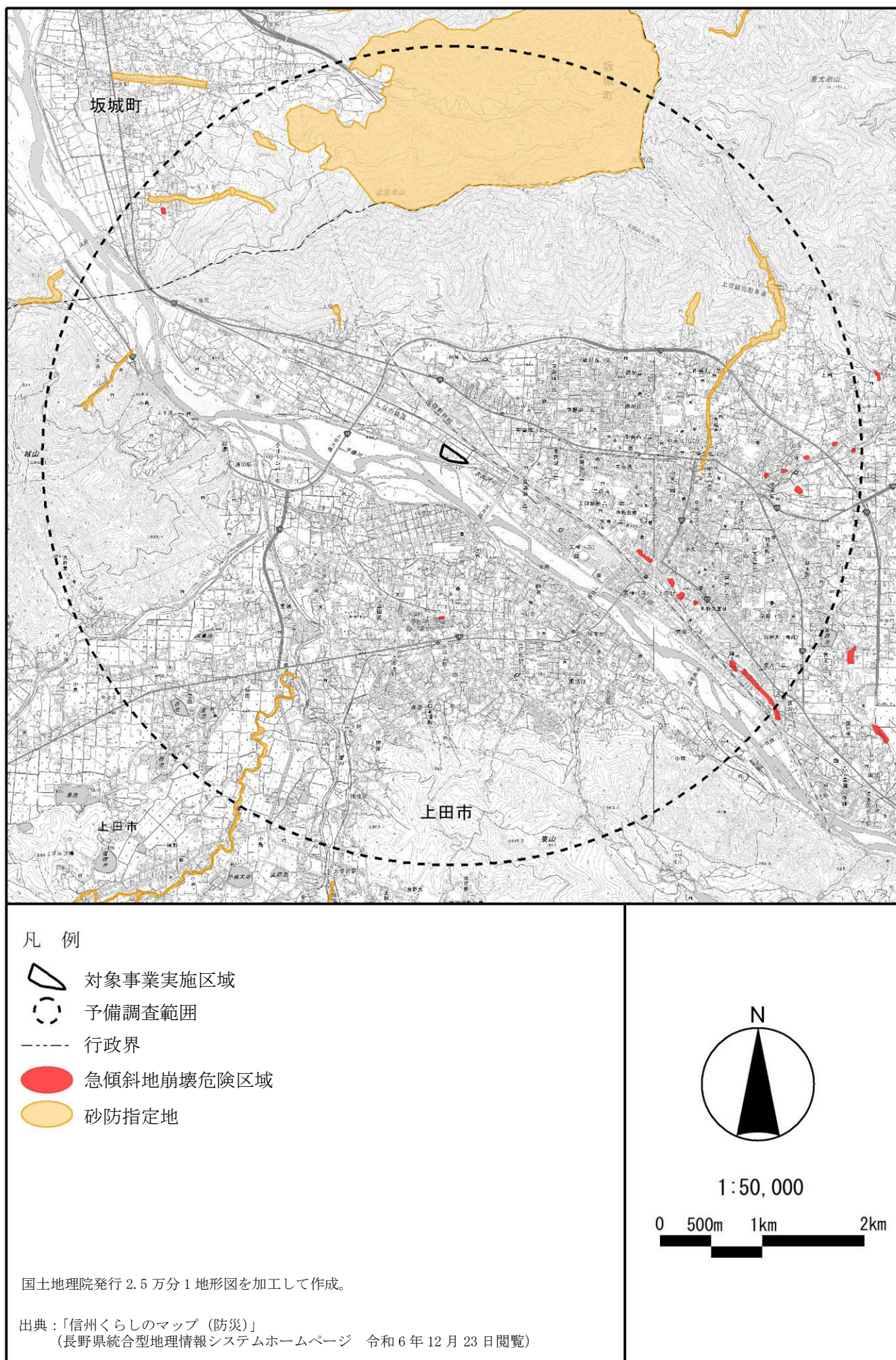
図 2.3-14 対象事業実施区域及びその周囲の砂防指定地、急傾斜地崩壊危険区域の指定状況
