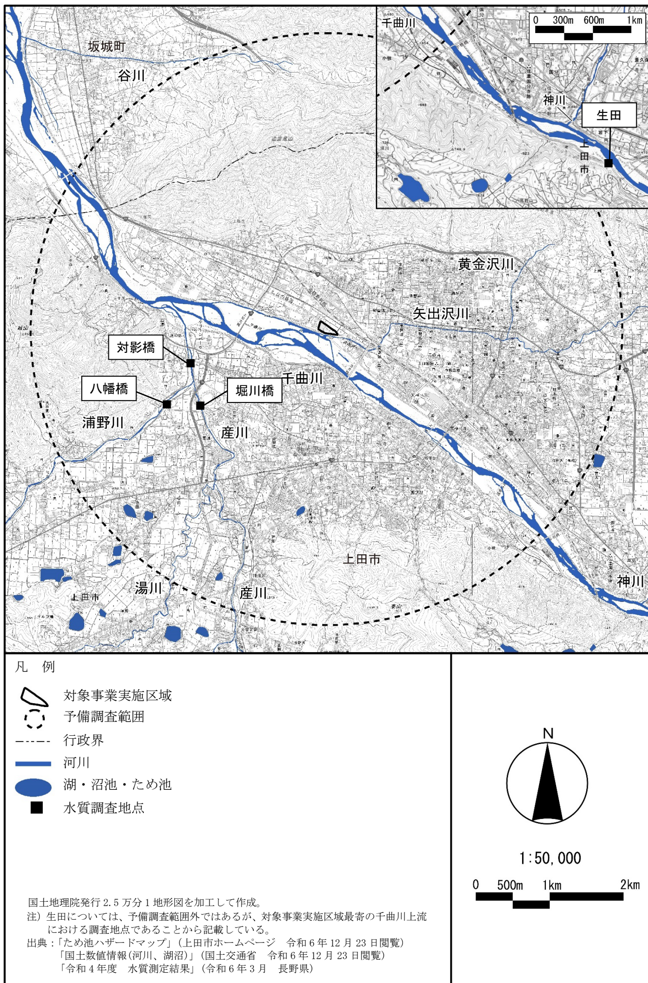
図 2.2-29 対象事業実施区域及びその周囲の河川の水質調査地点 1.2-75
