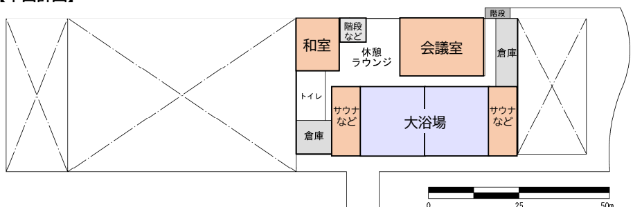
【平面計画】
